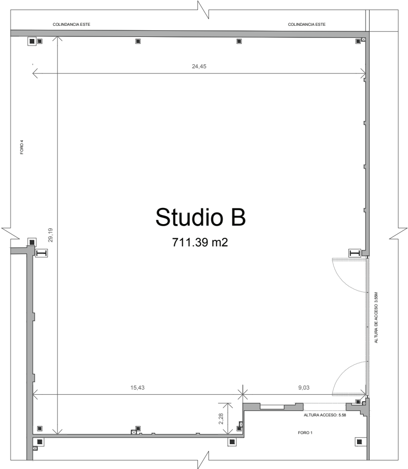
PLANTA ARQUITECTÓNICA
